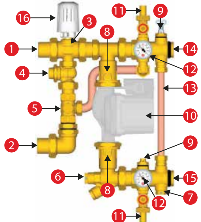
Составные элементы узла R557RY043
