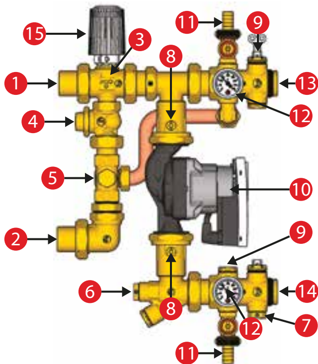
Составные элементы узла R557RY042
