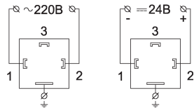
Схемы подключения катушки
