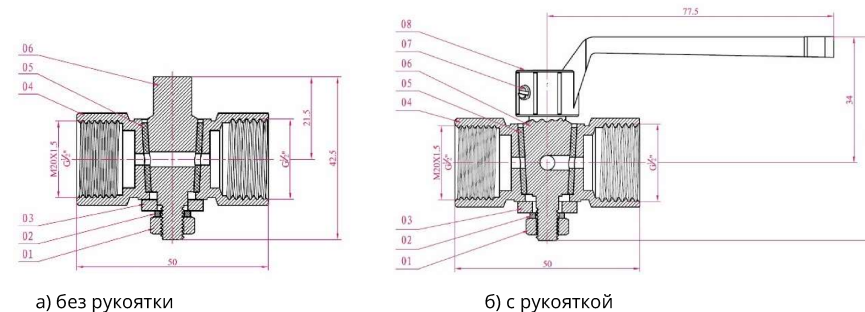
Рис.1 Кран 3-х ходовой 11Б18БК Ду 15 ВР G1/2"; G1/2"-M20x1,5.
