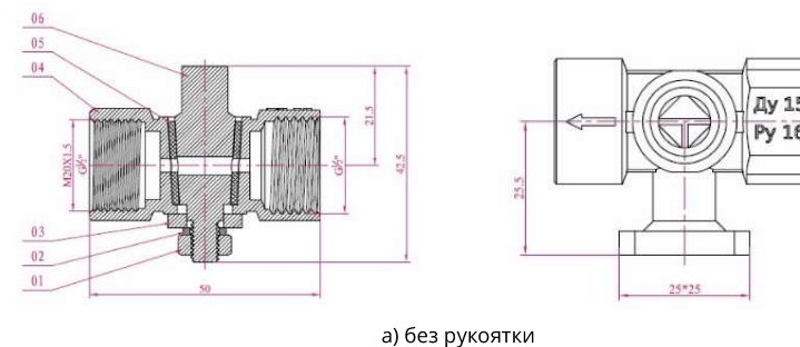
Рис.1 Кран 3-х ходовой 11Б18БК Ду 15 ВР G1/2"; G1/2"-M20x1,5.
