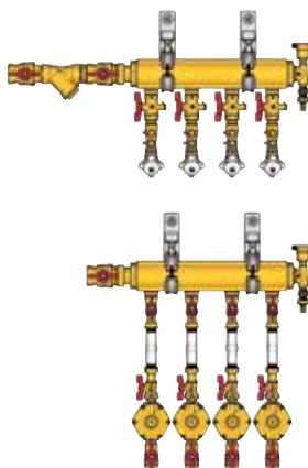
Коллекторы этажные с индивидуальной балансировкой системы отопления
