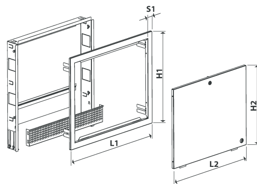
Сборочная схема и основные размеры шкафа R500
