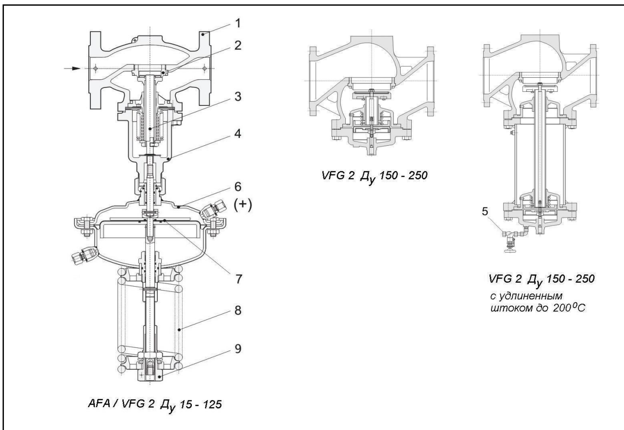
Рис. 3. Регулятор перепада давления AFA/VFG 2 (VFG 21).
