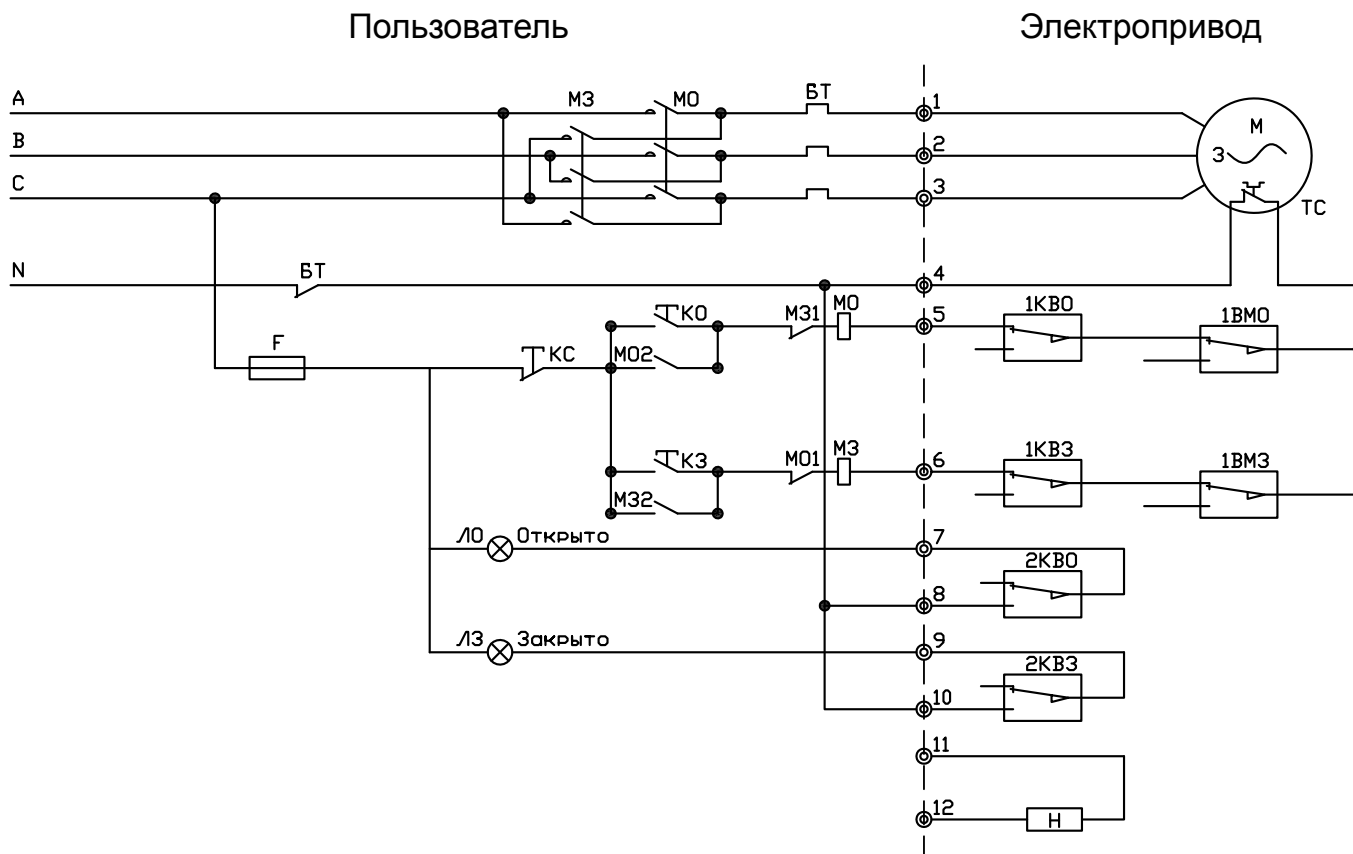
Рис. 3г. Принципиальная электрическая схема подключения электропривода ГЗ-ОФ(М) к сети 3 х 380 В, 50 Гц.
