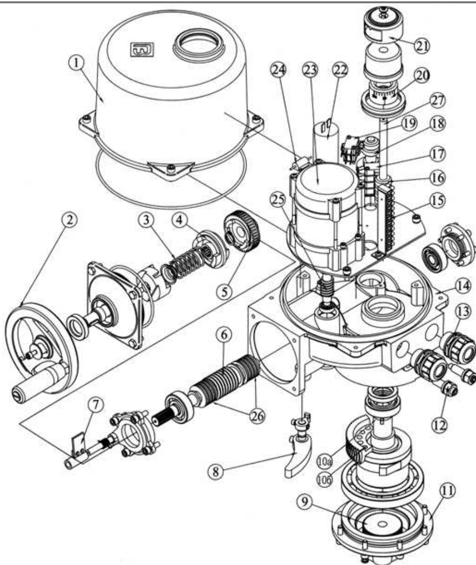
Рис.2 Электропривод ГЗ-ОФ(М)
