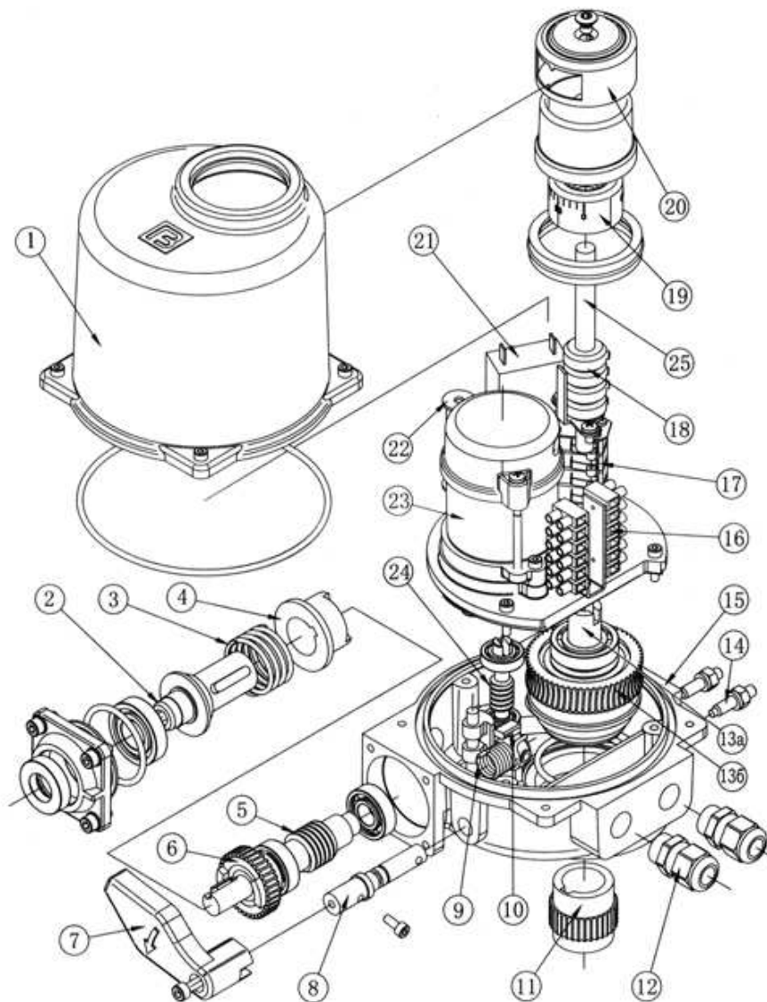
Рис.1 Электропривод ГЗ-ОФ(К)
