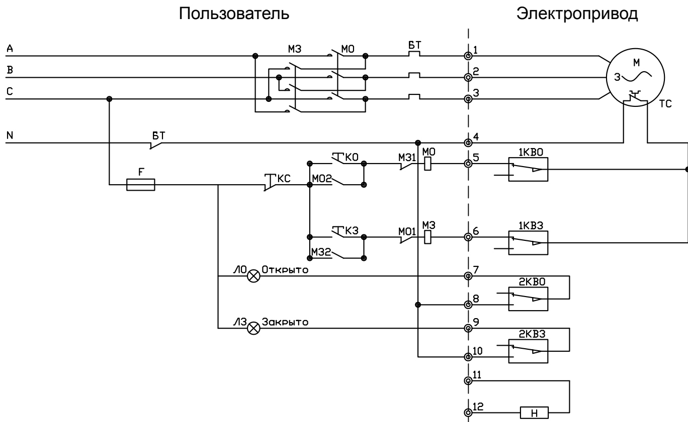
Рис. 3б. Принципиальная электрическая схема подключения электропривода ГЗ-ОФ(К) к сети 3 х 380 В, 50 Гц.
