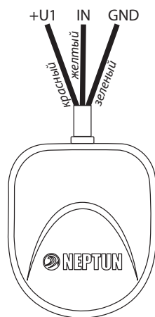
Рис. 7. Маркировка проводов.
