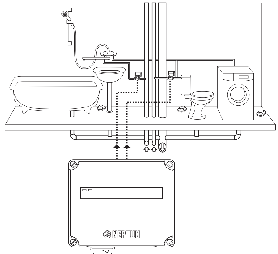
Рис. 4. Пример размещения комплекта в стандартной квартире.
