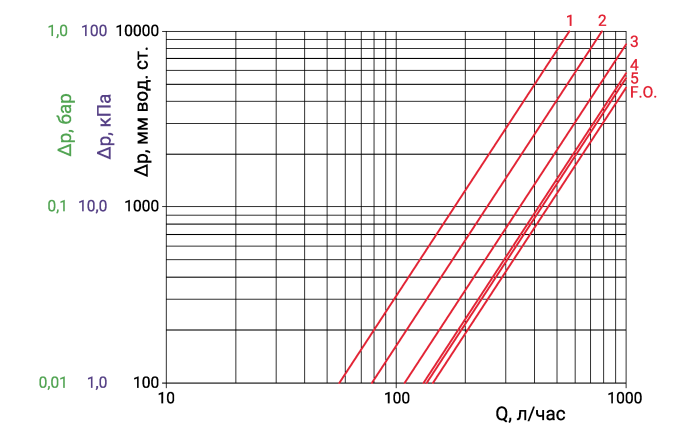
Значения пропускной способности для настройки клапанов коллектора R583S - R583V
